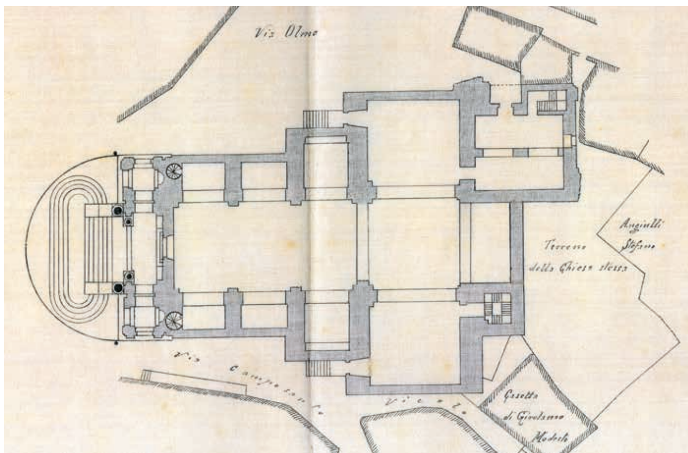
1913 - "Pianta attuale della Chiesa Comunale di Alberobello" - scala metrica 1/200
